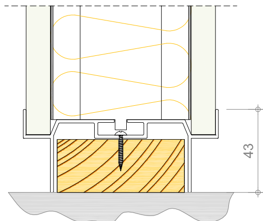
D vloer aansluiting
