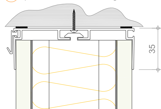
C plafond aansluiting
