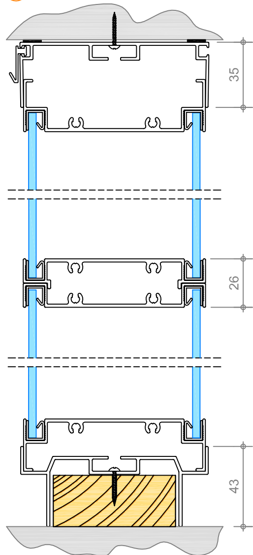
D vloer aansluiting
