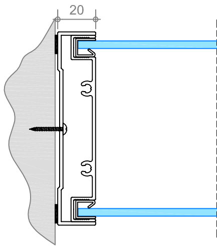
A vlakke wandaansluiting
