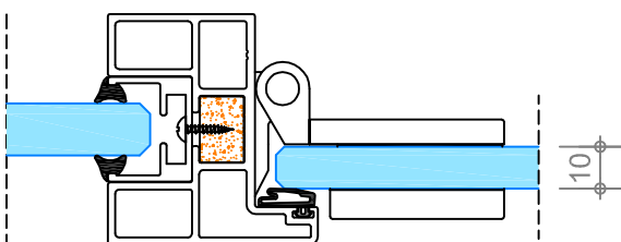
D horizontale doorsnede deurstijl
