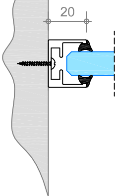
A vlakke wandaansluiting
