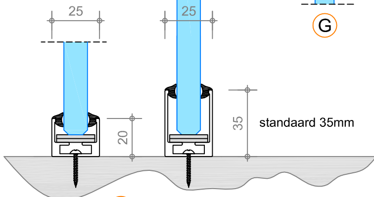
F vloer aansluiting
