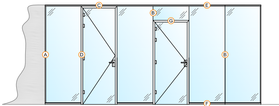
A vlakke wandaansluiting
