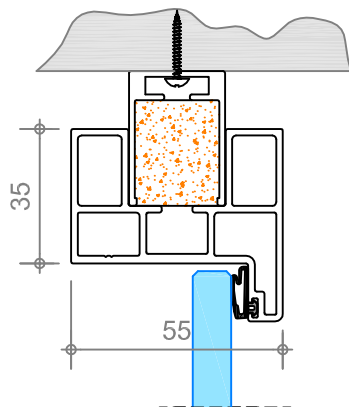
C plafondaansluiting deurkozijn
