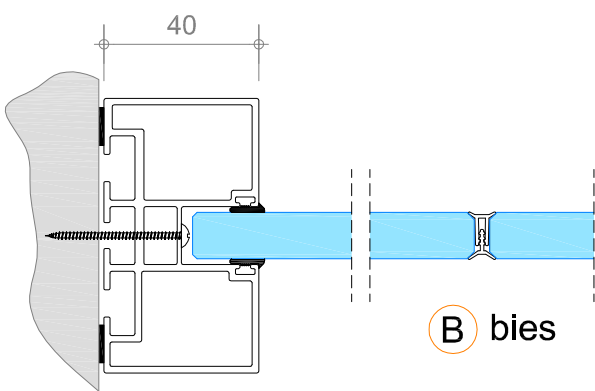
A vlakke wandaansluiting
