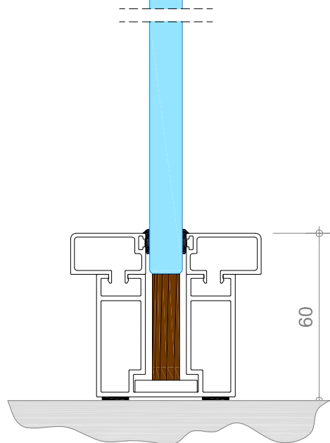
E vloer aansluiting
