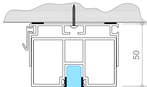
D plafond aansluiting
