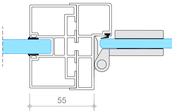
C verticale deurstijl
