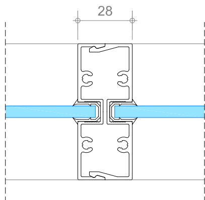
B verticale stijl
