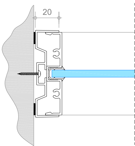
A vlakke wandaansluiting
