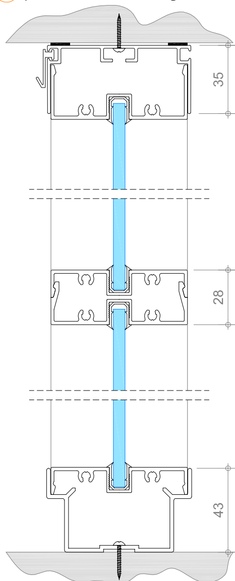
D vloer aansluiting
